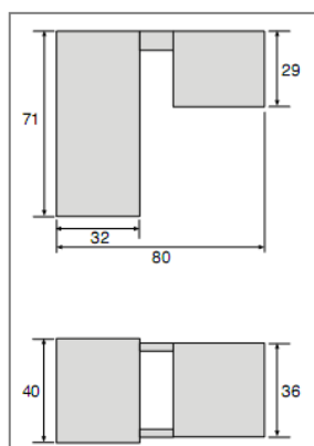
Monoblocco (cm. 40x80x71h)
